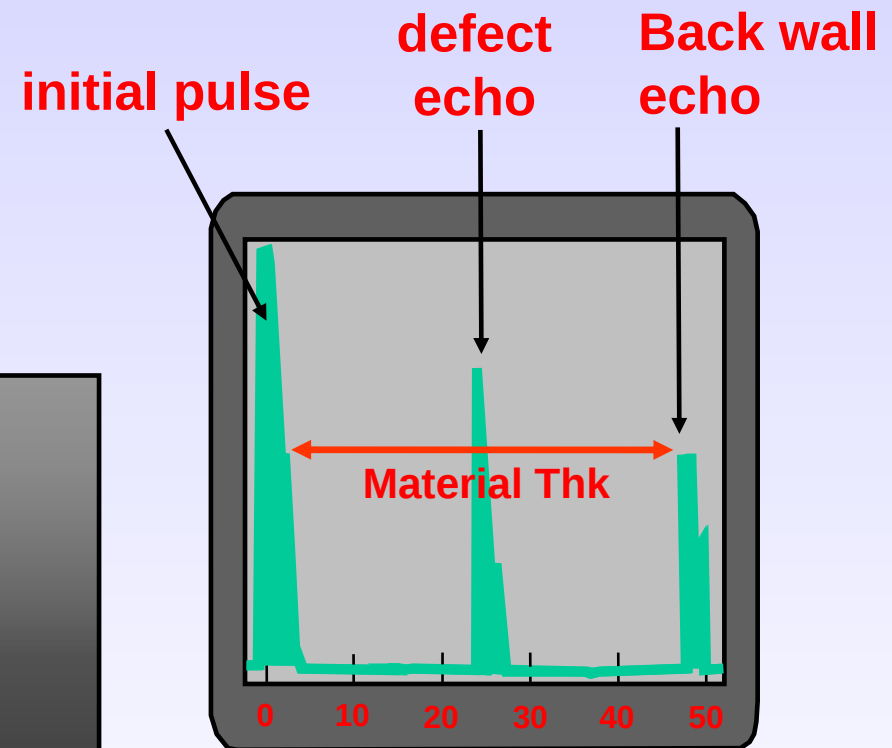
CRT Display
