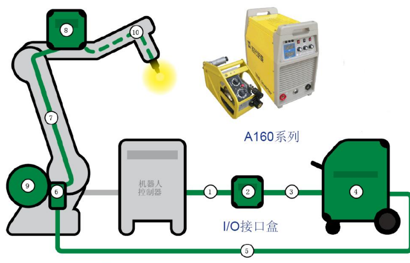
时代机器人焊接简易系统示意图
