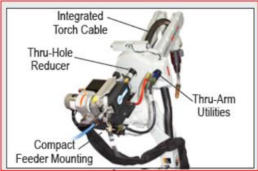
内置式集成设计
