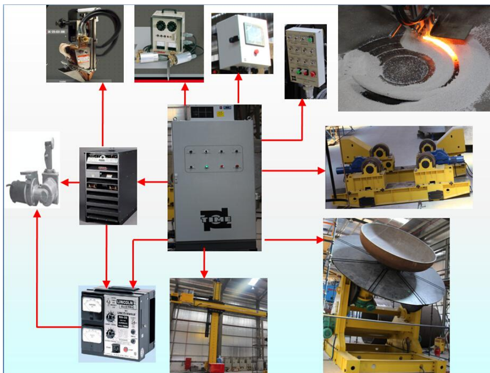
图 1：时代带极堆焊设备
