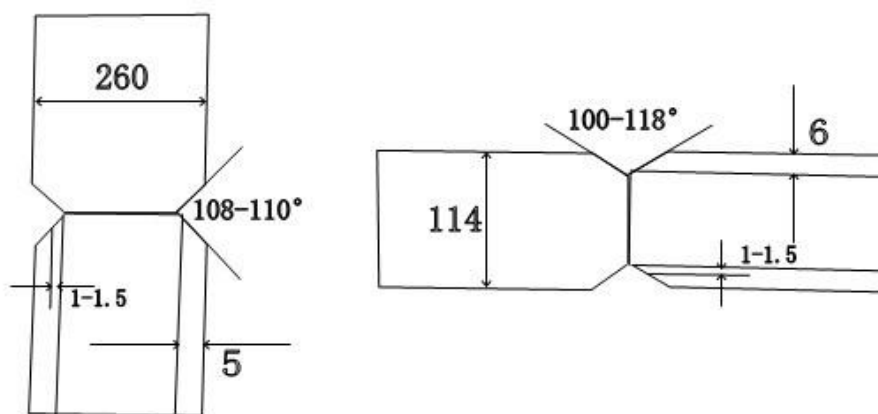
管对接垂直固定焊
